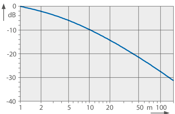
Abb. IV: Abnahme des Schalldruckpegels
