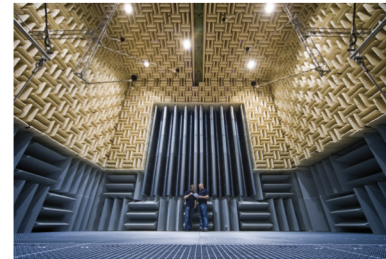
Abb. 1b: Prüfstand
