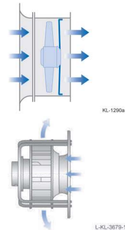
Einbauart A gemäß DIN ISO 5801
